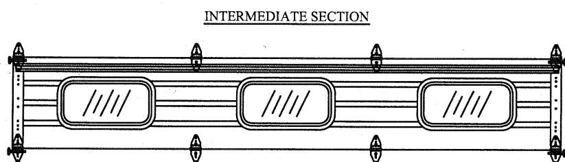
OPTIONAL GLAZED SECTION W/ 26" X 13" WINDOWS N.T.S.
