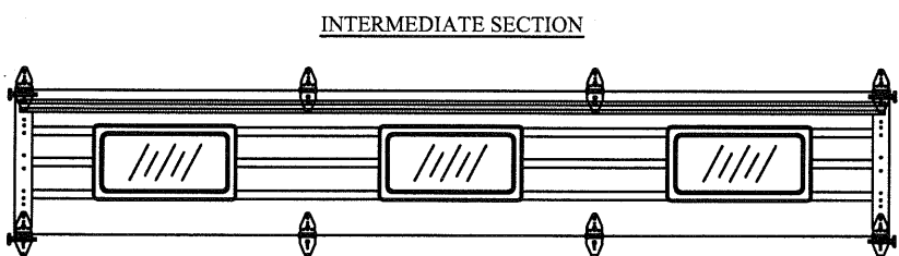
OPTIONAL GLAZED SECTION W/ 24" X 12" WINDOWS N.T.S.
