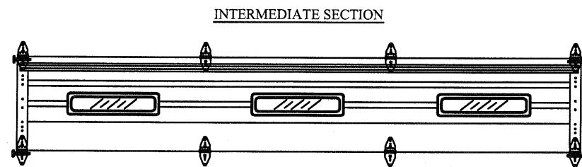
OPTIONAL GLAZED SECTION W/ 24" X 6" WINDOWS N.T.S.
